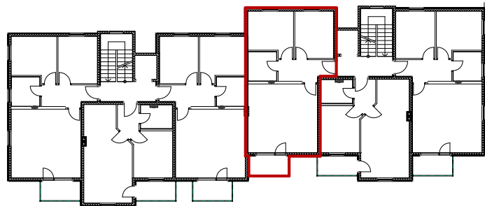
TLOCRT ETAŽE +1 - Pozicija stana na etaži
