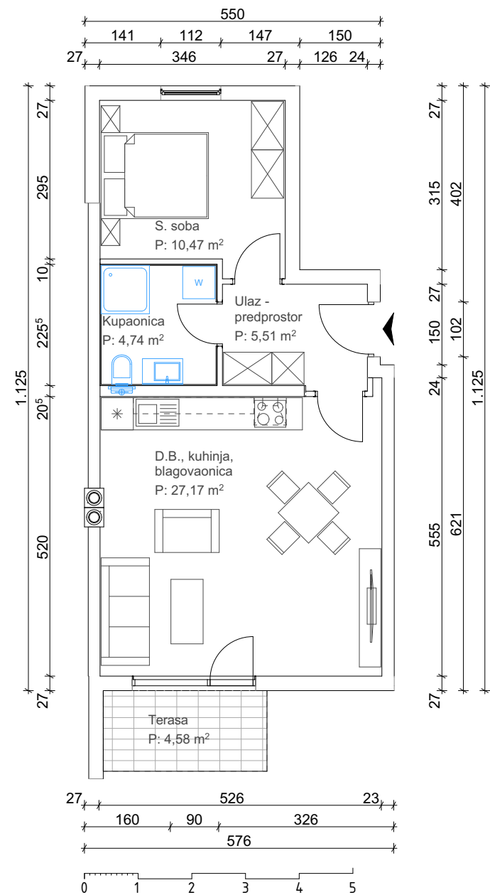
TLOCRT STANA
