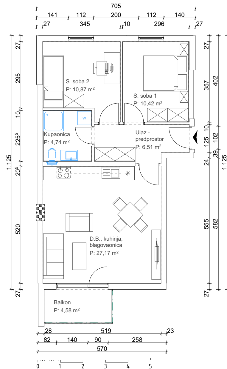
TLOCRT STANA
