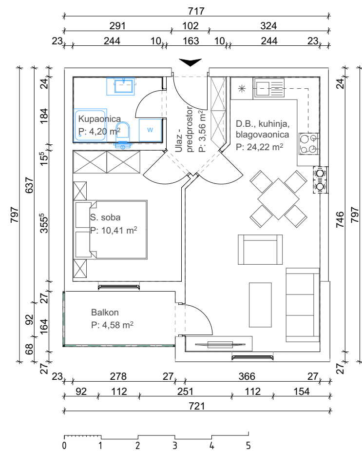
TLOCRT STANA
