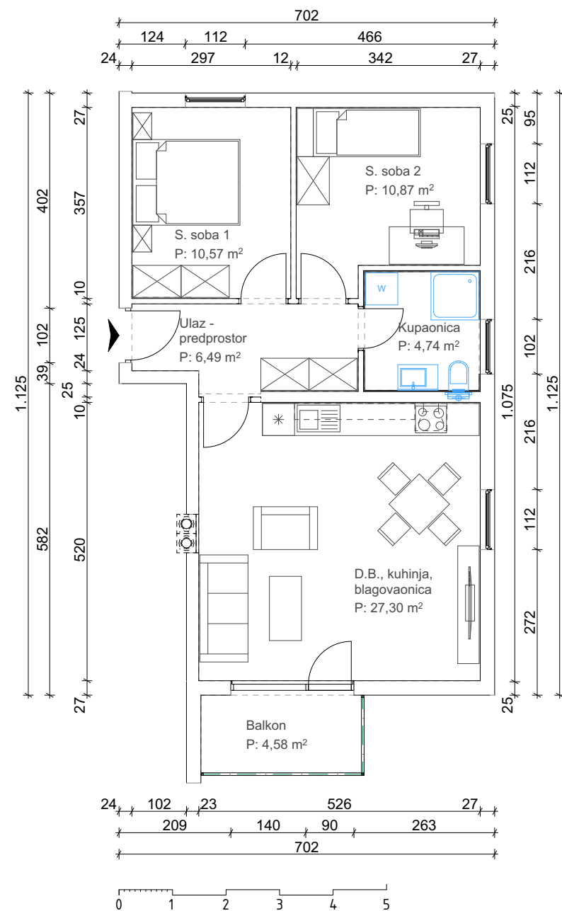
TLOCRT STANA
