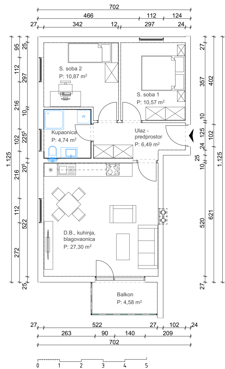
TLOCRT STANA
