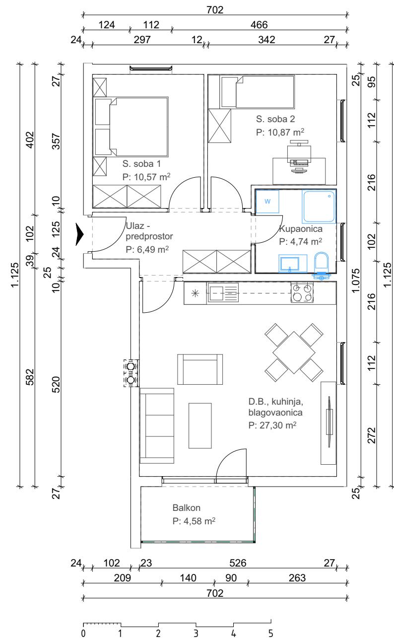
TLOCRT STANA
