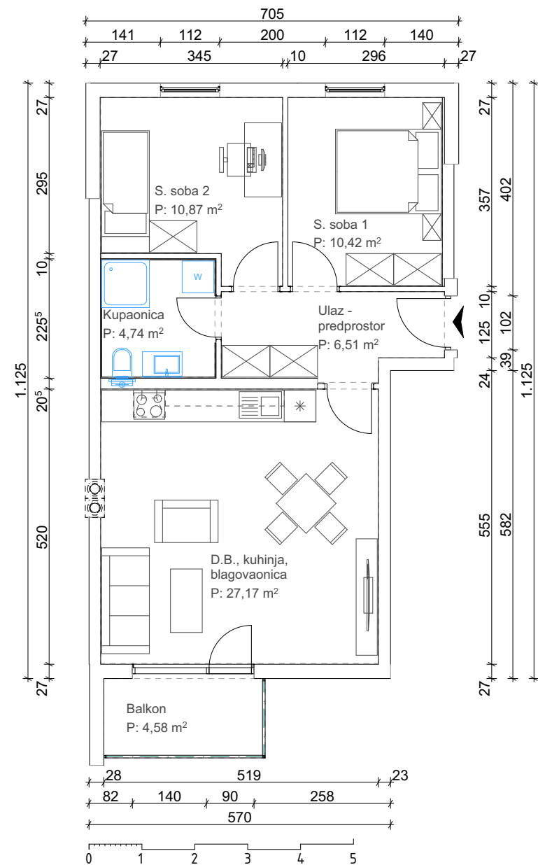
TLOCRT STANA
