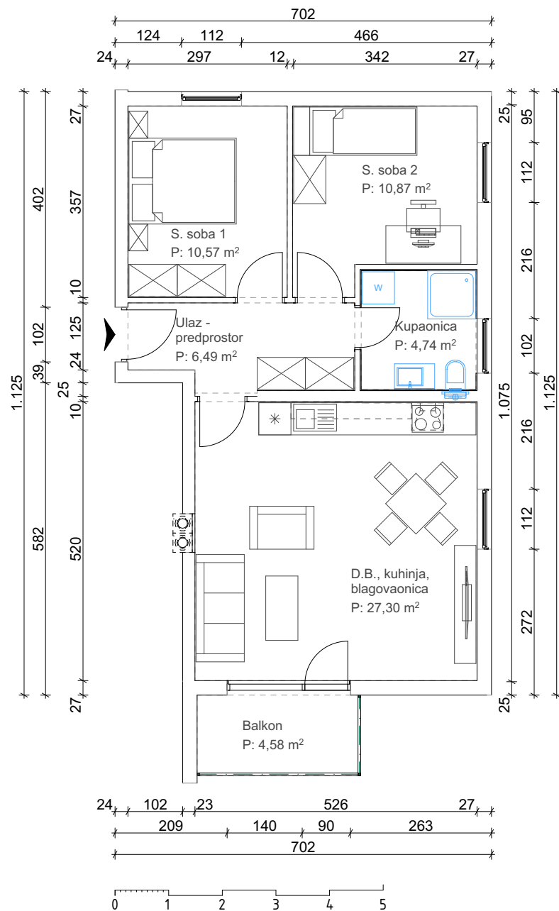
TLOCRT STANA
