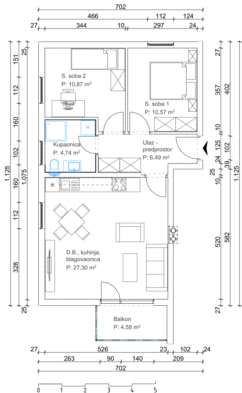
TLOCRT STANA
